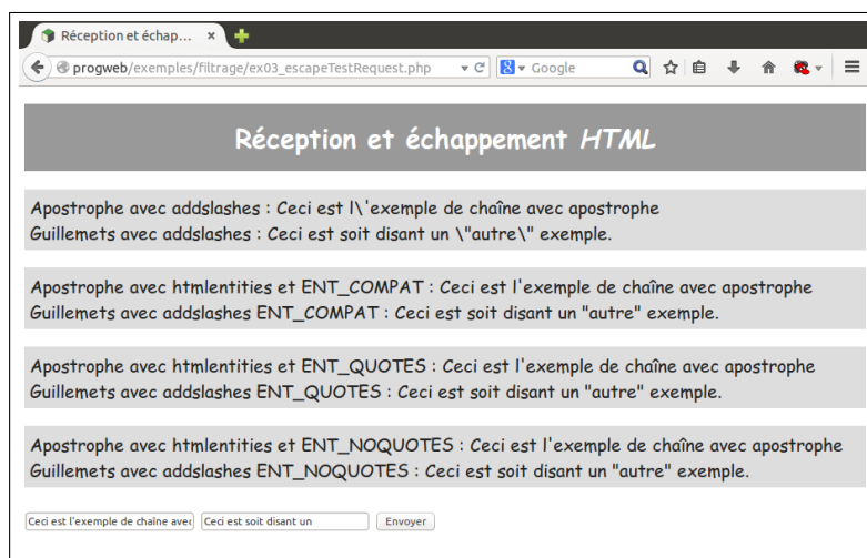
FIGURE 4.6 : Illustration du code source 4.5
