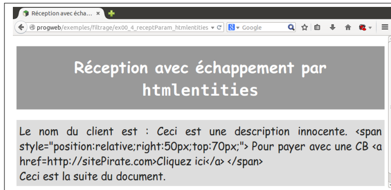
FIGURE 4.5 : L'injection a été évitée par échappement.
