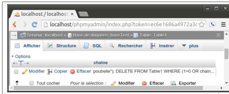
FIGURE 4.16 : Données dans la base après tentative d'injection SQL avec échappement
