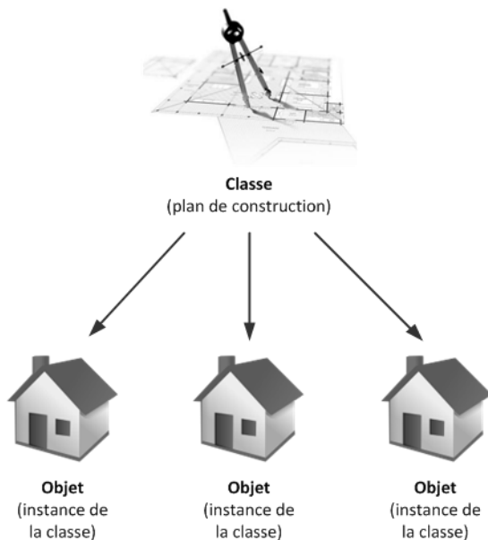
FIG. 27.4 – Classes et objets
