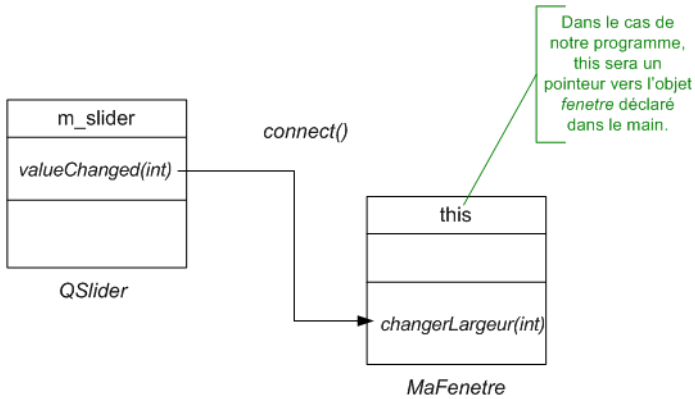
FIGURE 24.10 – Connexion entre le slider et la fenêtre
