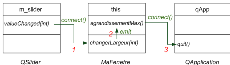
FIGURE 24.13 – Échange de signaux entre objets
