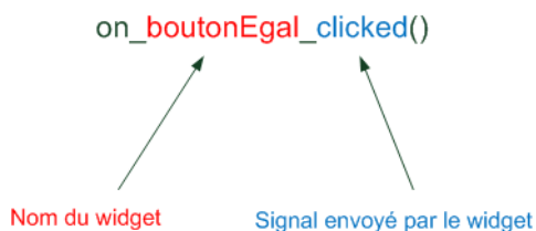
FIGURE 31.18 – Donnez un nom précis à votre slot et la connexion sera automatique!
