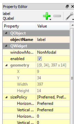
FIGURE 31.10 – Éditeur de propriétés
