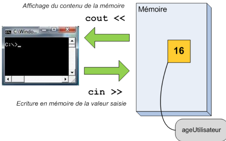
FIGURE 5.1 – Schéma mnémotechnique indiquant le sens à utiliser pour les chevrons
