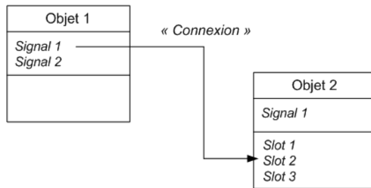
FIGURE 24.2 – Des signaux et des slots
