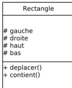
FIGURE 40.1 – Modélisation de la classe Rectangle
