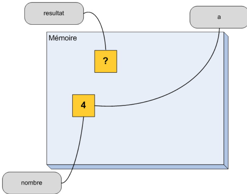
FIGURE 7.6 – État de la mémoire dans la fonction après un passage par référence
