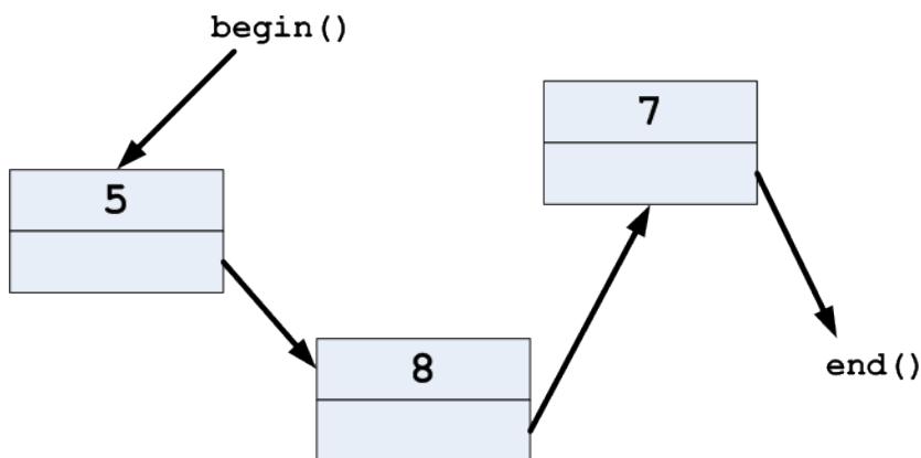
FIGURE 35.1 – Une liste chaînée ( list )
