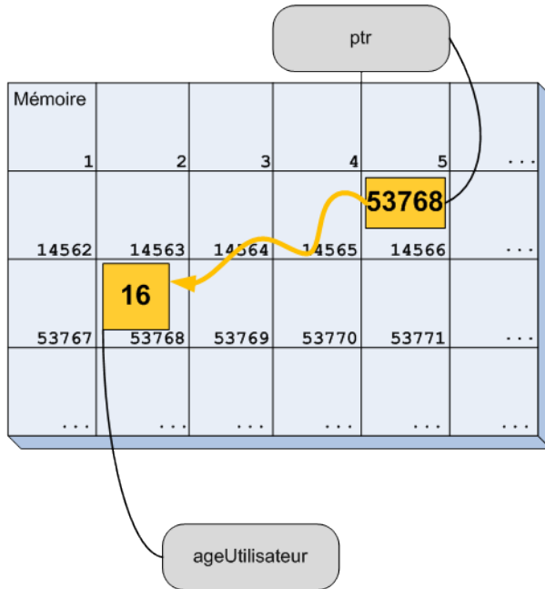
FIGURE 11.3 – La mémoire après la déclaration d’une variable et d’un pointeur pointant sur cette variable
