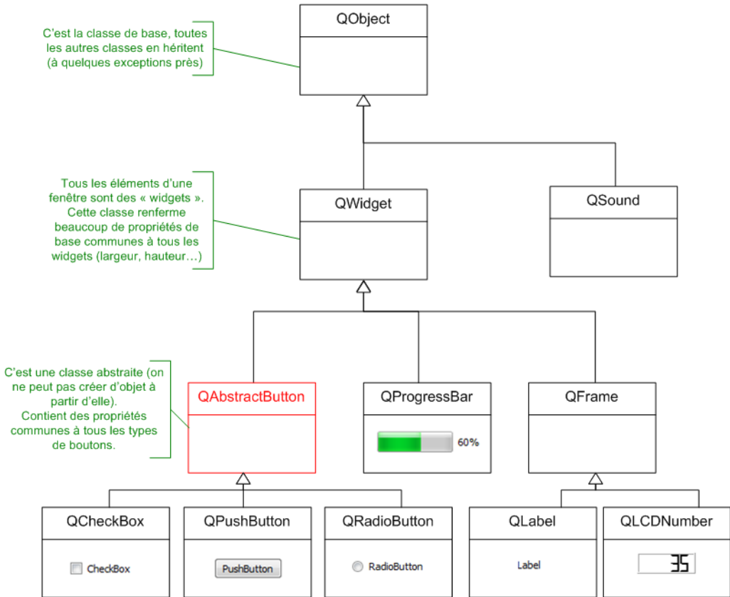
FIGURE 23.9 – Héritage sous Qt
