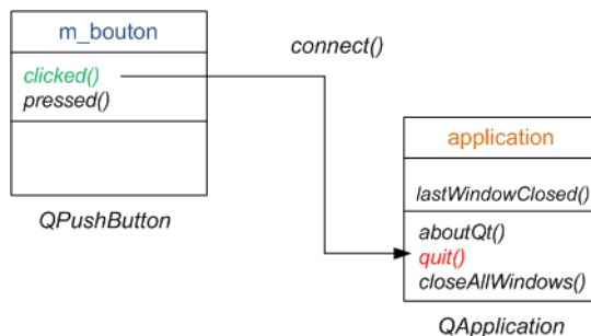
FIGURE 24.3 – Signaux et slots en pratique
