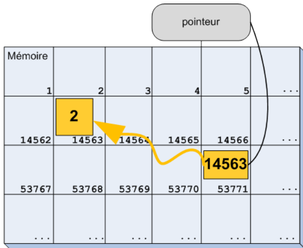
FIGURE 11.5 – La mémoire après avoir alloué une variable et changé la valeur de cette variable
