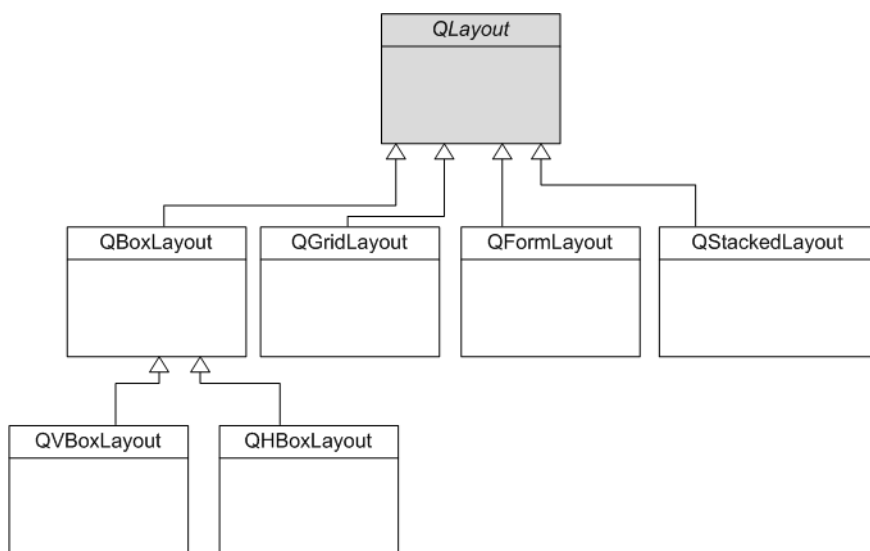
FIGURE 27.3 – Layouts avec Qt
