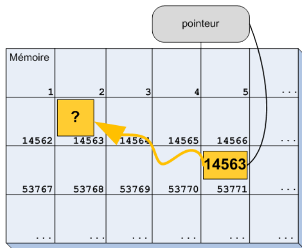
FIGURE 11.4 – La mémoire après l'allocation dynamique d'un entier
