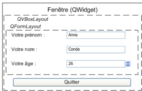
FIGURE 27.19 – Schéma des layouts combinés
