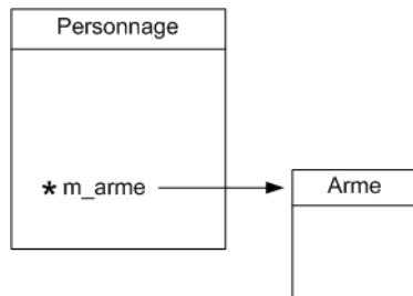
FIGURE 17.2 – Des classes liées par un pointeur
