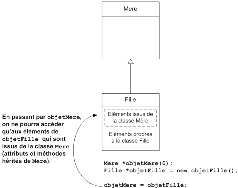
FIGURE 18.4 – La dérivation de type
