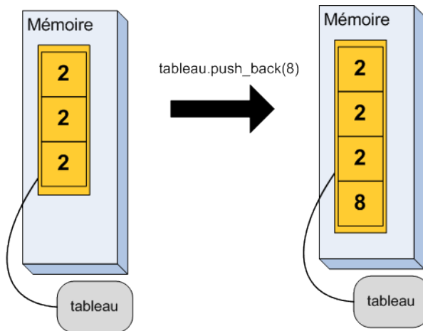
FIGURE 8.4 – Effet d'un push_back sur un vector
