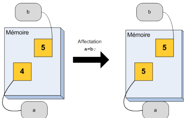
FIGURE 5.2 – Affectation d'une variable à une autre
