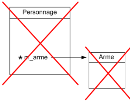
FIGURE 17.4 – Tous les objets sont proprement supprimés
