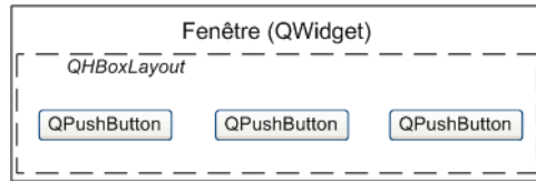
FIGURE 27.7 – Schéma des layouts
