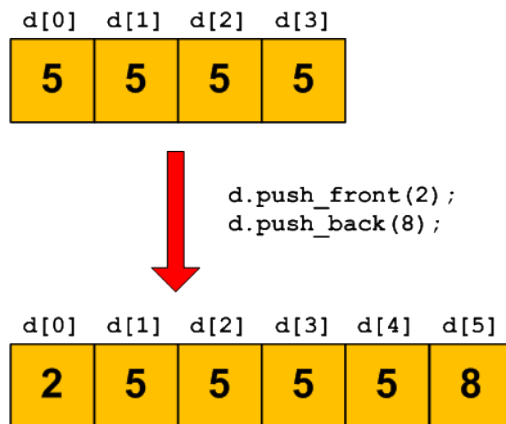
FIGURE 34.1 – Fonctionnement d'une deque
