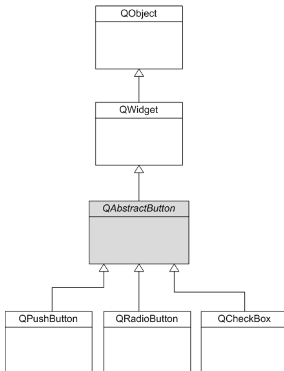
FIGURE 28.7 – L’héritage des boutons
