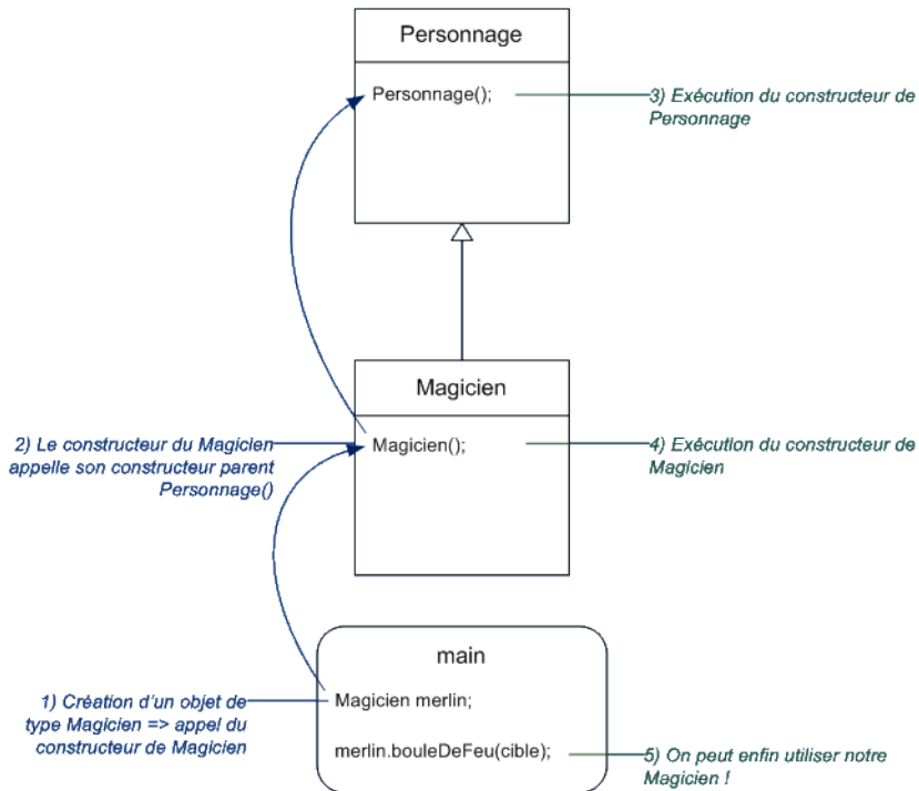
FIGURE 18.5 – Ordre d'appel des constructeurs
