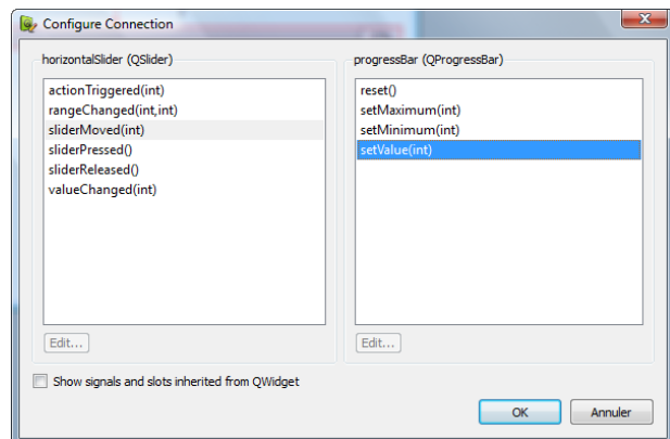
FIGURE 31.13 – Choix des signaux et slots
