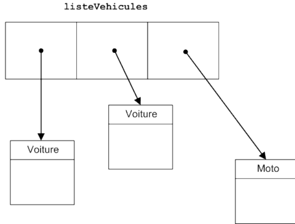
FIGURE 19.2 – Une collection hétérogène
