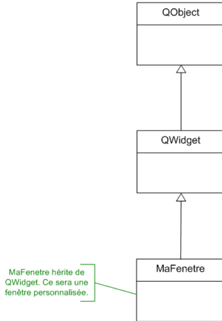
FIGURE 23.14 – MaFenetre hérite de QWidget
