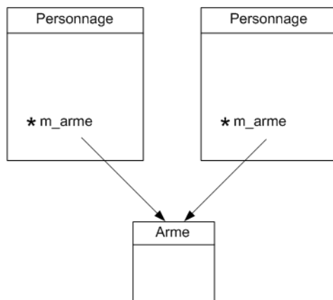
FIGURE 17.6 – L’ordinateur a copié le pointeur, les deux Personnages pointent vers la même Arme
