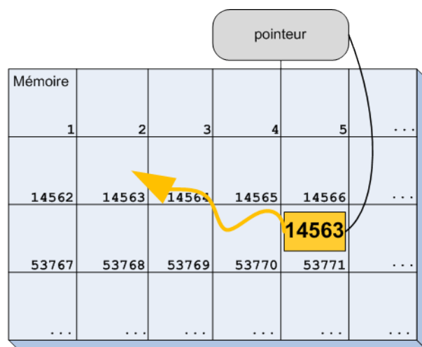
FIGURE 11.6 – Un pointeur pointant sur une case vide après un appel à delete
