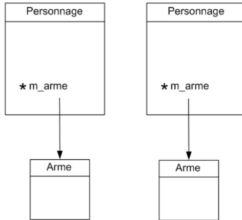
FIGURE 17.7 – Chaque personnage a maintenant son arme
