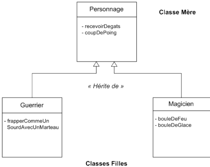
FIGURE 18.2 – Deux classes héritent d’une même classe
