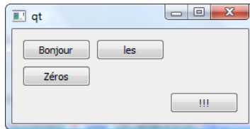
FIGURE 27.12 – Bouton en bas à droite
