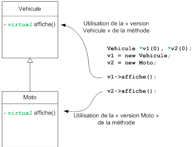
FIGURE 19.1 – Fonctions virtuelles et pointeurs
