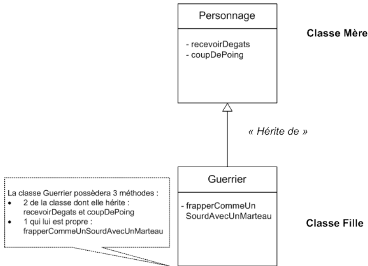
FIGURE 18.1 – Un héritage entre classes
