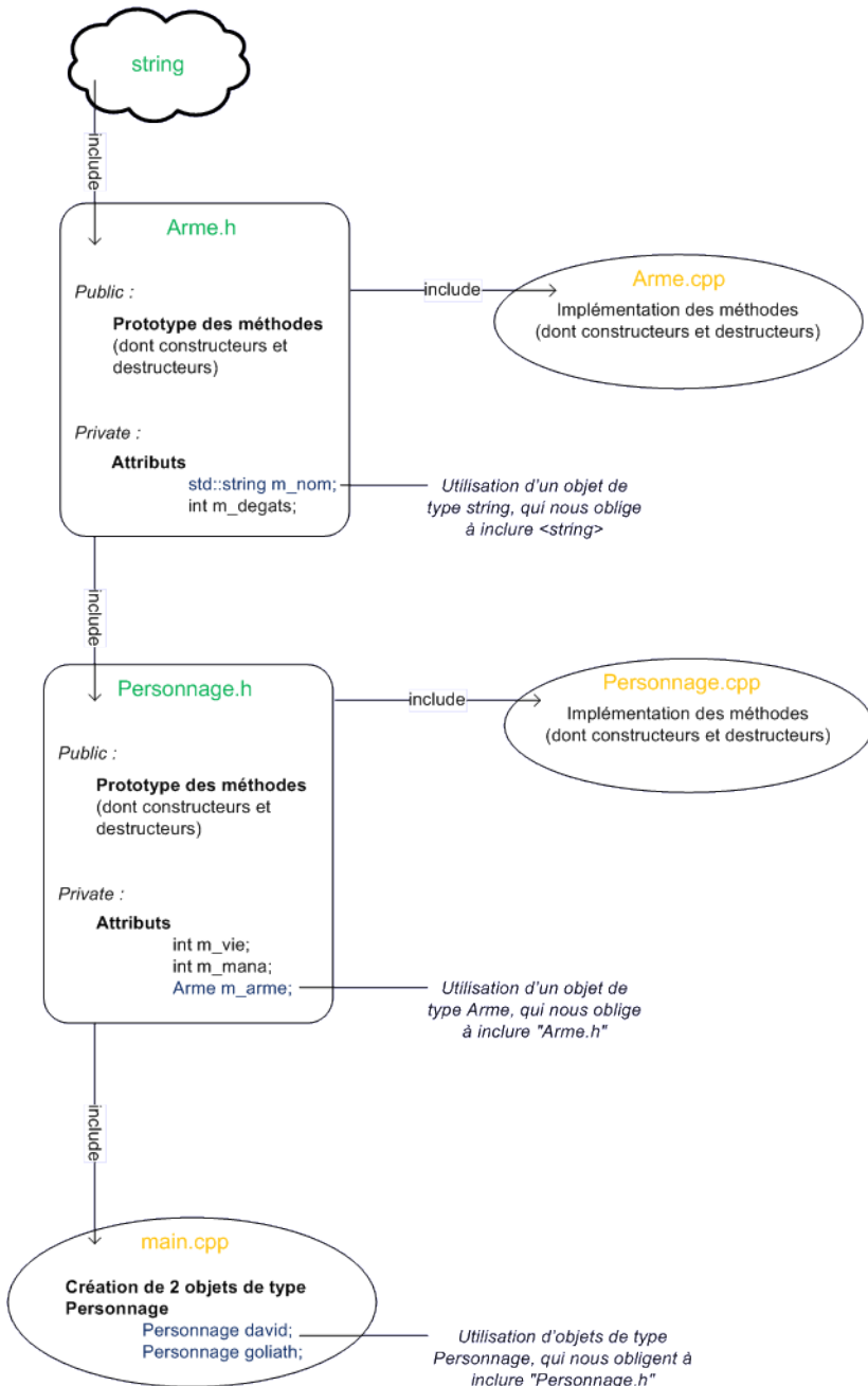
FIGURE 14.1 – Résumé de la structure du code
