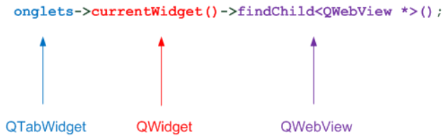
FIGURE 32.5 – Utilisation de findChild
