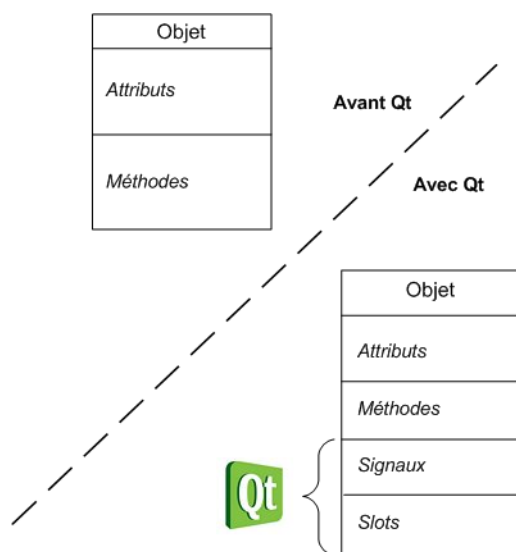
FIGURE 24.1 – Un objet avec des signaux et des slots
