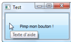
FIGURE 23.3 – Une infobulle
