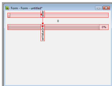
FIGURE 31.14 – Connexion établie !
