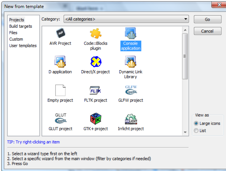
FIGURE 2.4 – Nouveau projet
