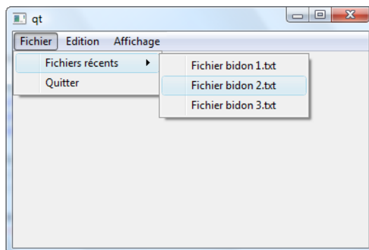
FIGURE 30.8 – Les sous-menus
