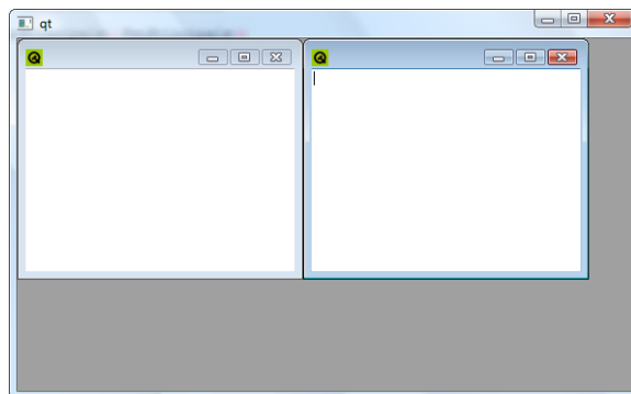
FIGURE 30.5 – Des sous-fenêtres
