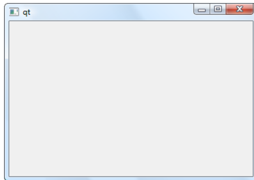
FIGURE 28.1 – Fenêtre vide
