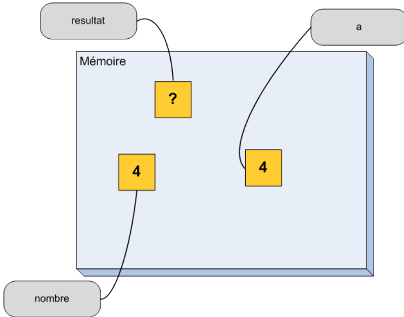
FIGURE 7.5 – État de la mémoire dans la fonction après un passage par valeur
