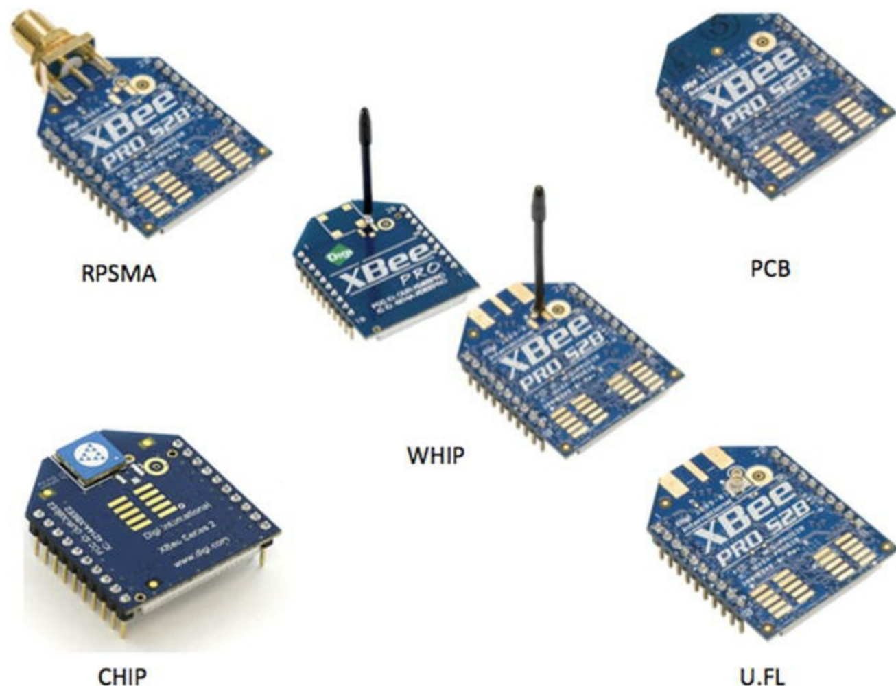
Figure 2-1. XBee module antenna options
