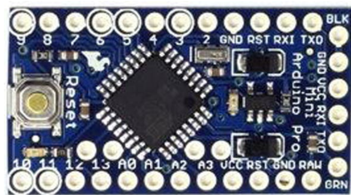
Figure 3-9. Arduino Pro Mini (courtesy of Arduino.cc)
