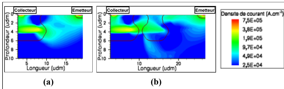
Figure 138: Distributions de densité de courant dans la structure de référence au point TLP ( V=32,1\text{ V} ; I=1,54\text{ A} ) (a), et dans la structure de distance 0,9 \mu\text{dm} au point TLP ( V=54,6\text{ V} ; I=1,49\text{ A} ) (b).
