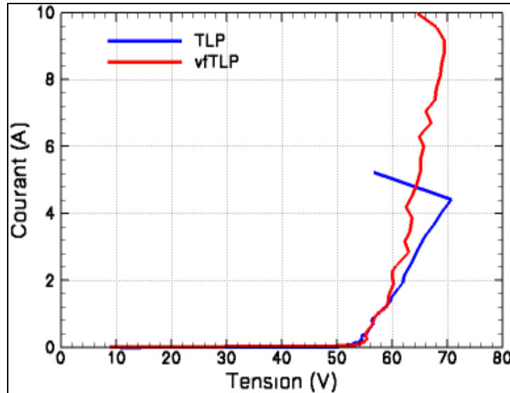
Figure 80: Comparisons des caractéristiques TLP et vfTLP mesurées pour le composant DUT4.
