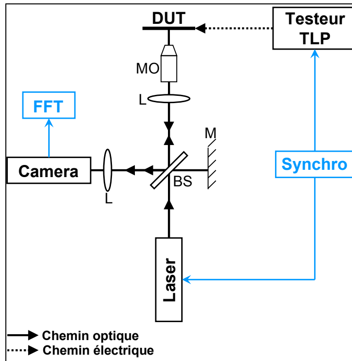
Figure 16: Schéma de principe de la méthode TIM (M : Miroir, L : Lentille, MO : Objectif de microscope, BS : Séparateur de faisceau).
