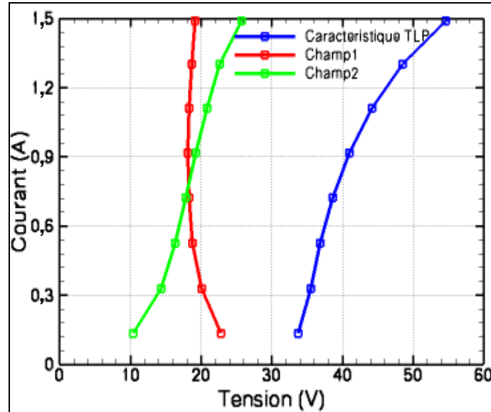
Figure 136: Caractéristique TLP fort courant et courbes I-V des contributions "Champ1" et "Champ2".
